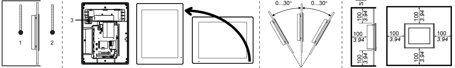
1 Internal temperature/ 盤内温度 /Température interne/Innentemperatur/Temperatur interna/Temperatur interna/ 内部温度 2 External temperature/ 盤外温度 /Température externe/Außentemperatur/Temperatur externa/Temperatur esterna/ 外部温度 3 Power connector/ 電源コネクタ /Connecteur d'alimentation/Netzanschluss/Conector de alimentación/Connettore di alimentazione/ 电源接头
